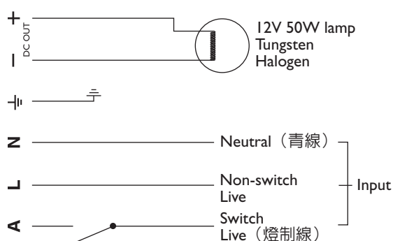
Maintained Type 長明式
