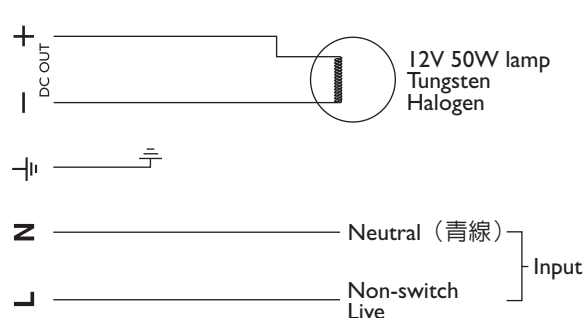
Non-maintained Type 後備式
